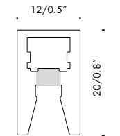
montantelettrico ma1 scala · scale 1:1
